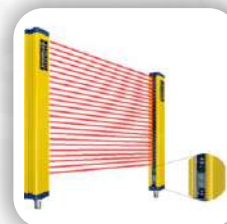
Grau de proteção Ip67 ou Ip69k. Tamanhos de 160mm a 1660mm. Distâncias funcionamento 2 a 20m. Vários acessórios disponíveis.
