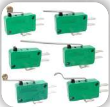
Micro chave 1 reversível com diversos atuadores.
